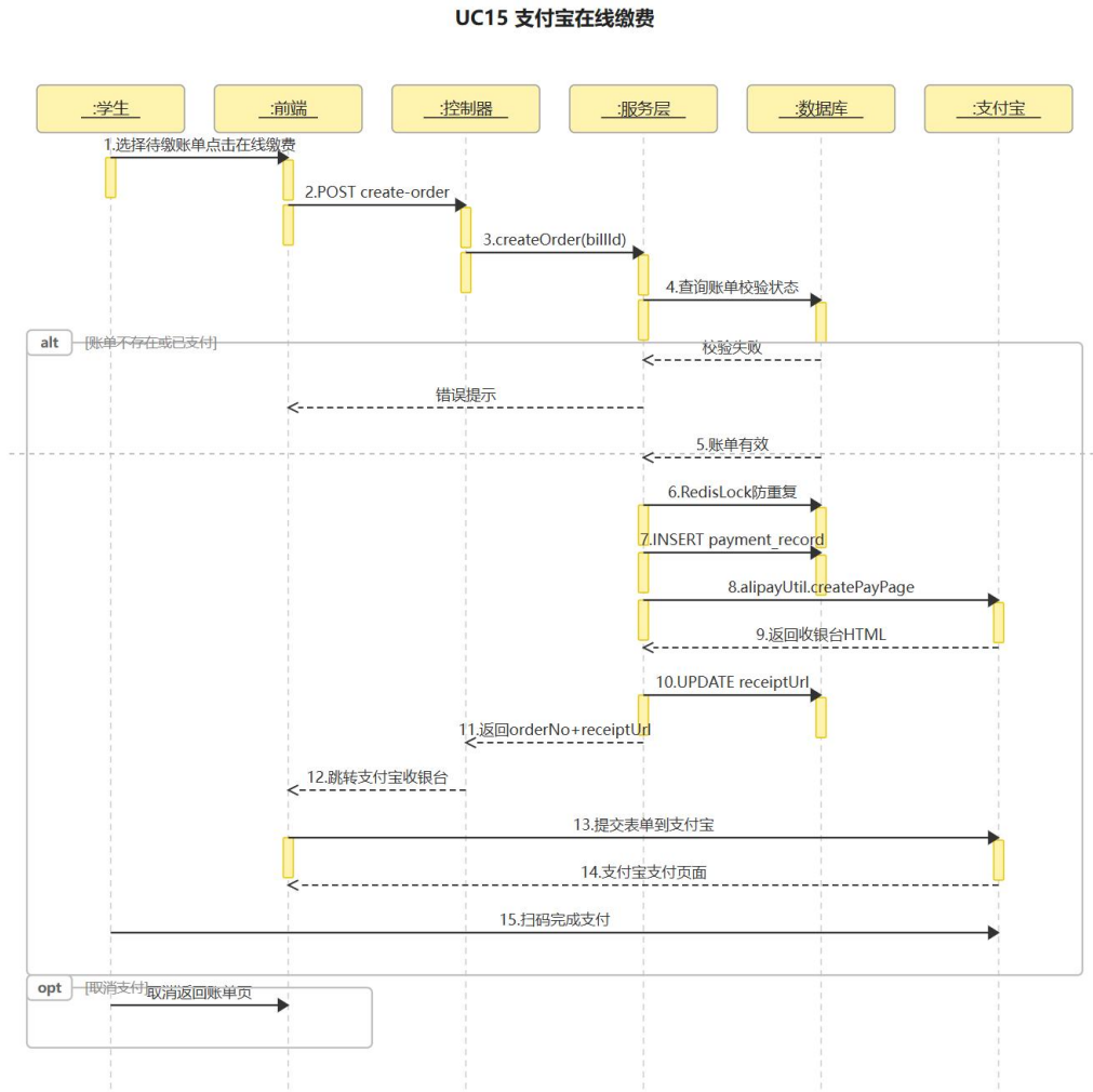
图 5-6 UC15 支付宝在线缴费用例顺序图
