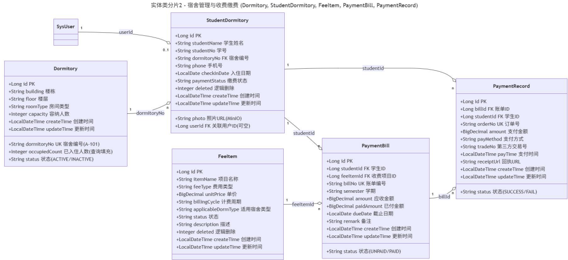
图 3-2 实体类图二
