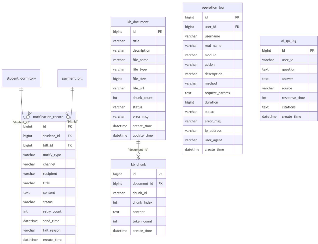
图 4-2 数据库关系图二
