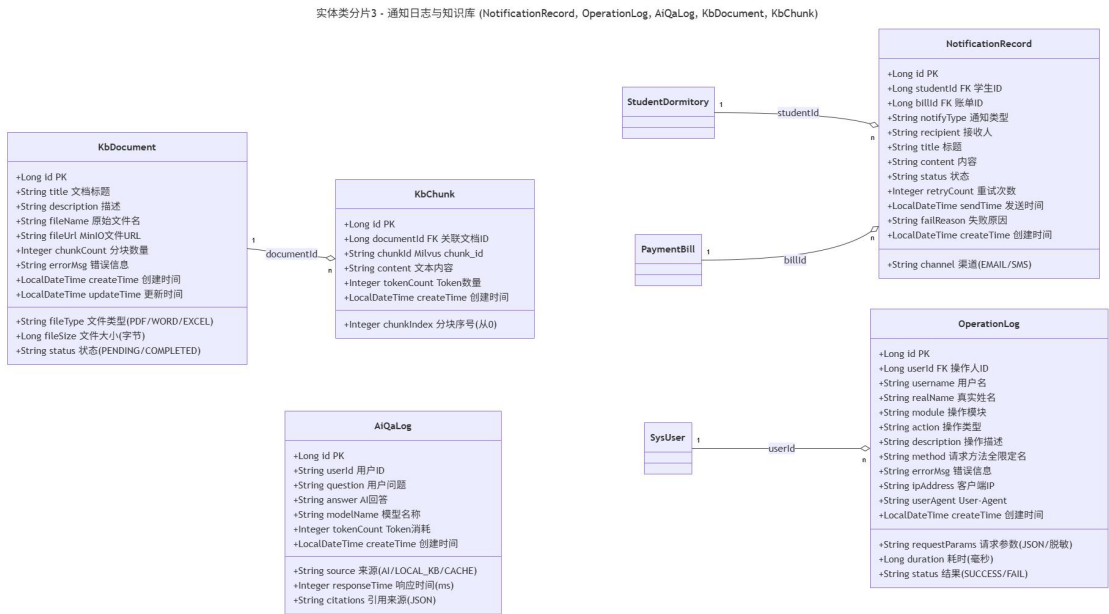
图 3-3 实体类图三
